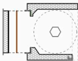
CK-4 TAGLIO DI MITA
