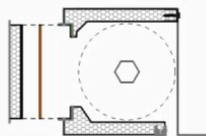
CK-3 CON LAMIERA PIÙ PORTA CAPPOTTO
